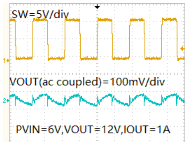
VOUT 纹波(PVIN=6V, VOUT=12V, IOUT=1A)
