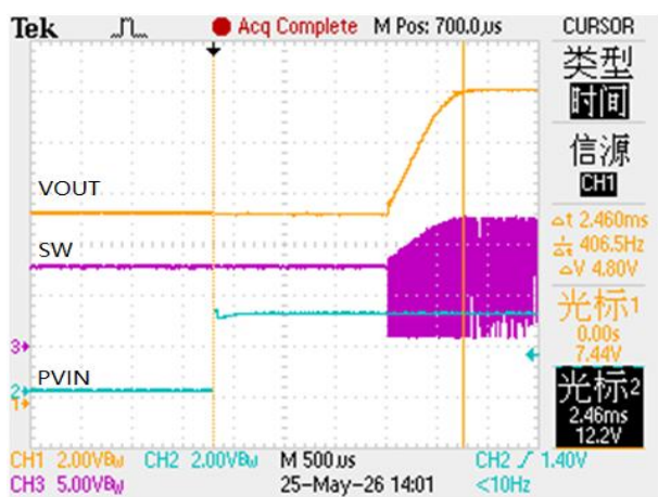
启动时间(7.4V 升 12V)
