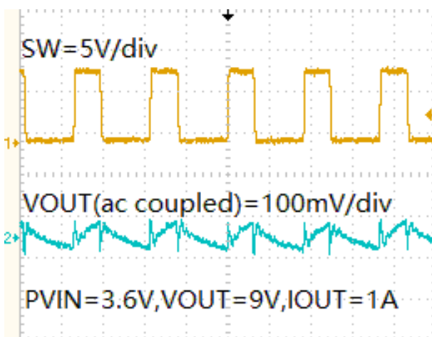
VOUT 纹波(PVIN=3.6V,VOUT=9V,IOUT=1A)
